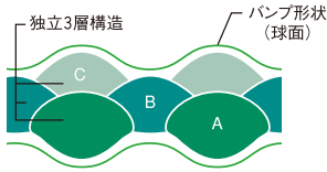
独立3層式バンブ構造
